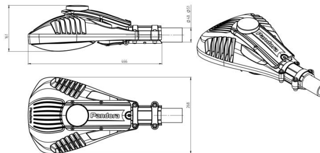
Рисунок 3. Габаритный чертеж.
